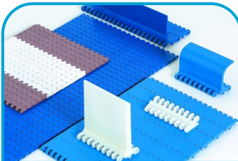
MODÜLER BANTLAR
