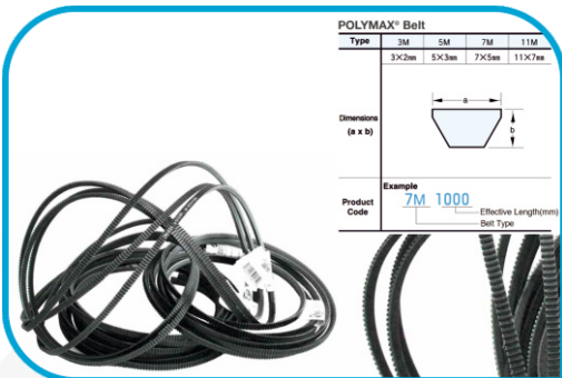
POLYMAX V KAYIŞI
